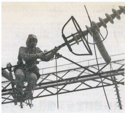
《云南电力报》 1997年9月19日 总第154期一期 滇中电业杯 为确保十五大期间工农业生产用电和城市居民生活用电，滇中电业局坚持多供少用的原则，用带电作业的形式对三岔站220千伏母线进行更换，取得了良好的经济效益和社会效益。图为9月1日14时带电作业时的情景。 (赵万波 摄)
