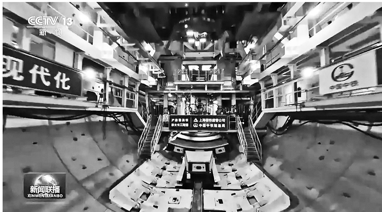
“领航号”盾构机在崇太长江隧道掘进施工
